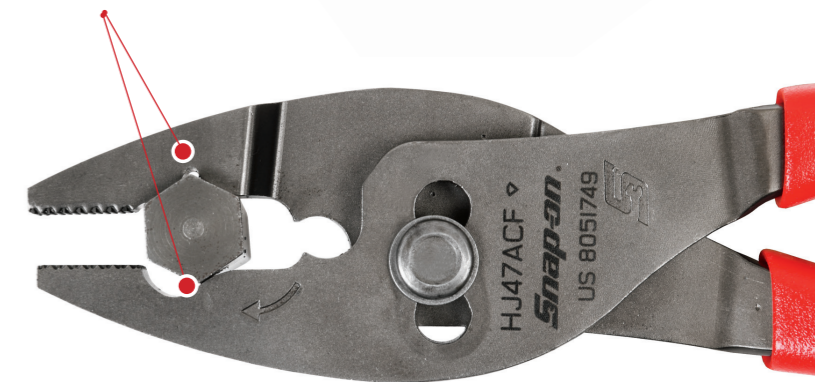
"Flankjaw" - Greifen von Muttern oder Bolzen auf der Flanke 30% mehr Drehkraft
